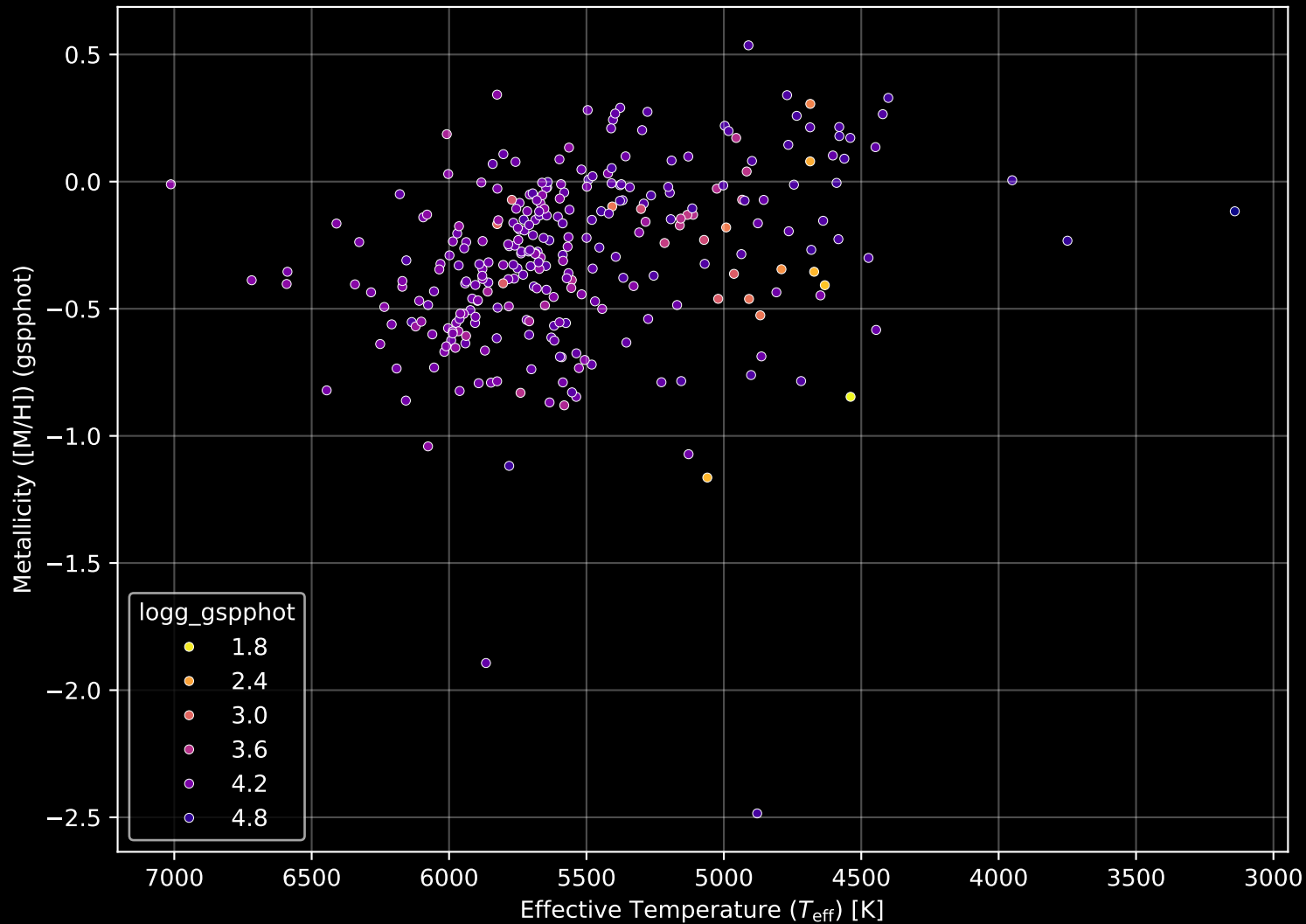
GALAH DR4 Field: [6890] Stellar Population Parameters (n= 293)
